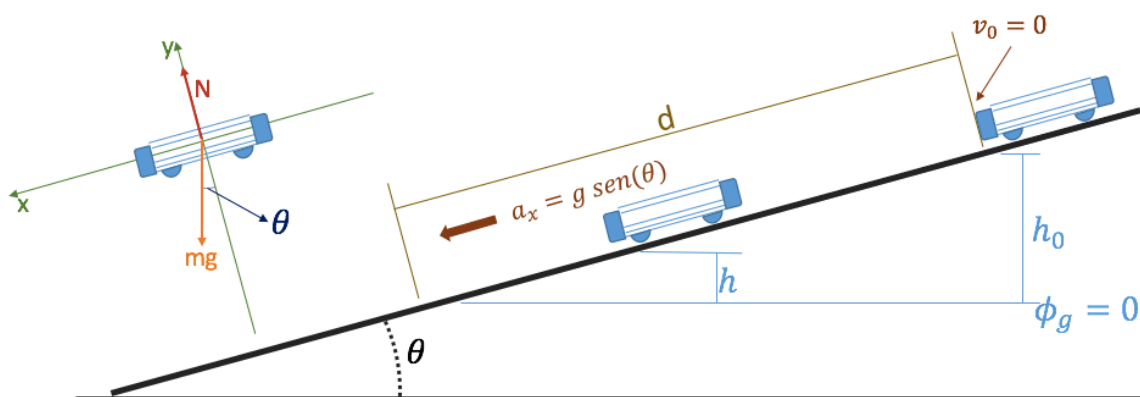
Figura 1. Esquema del plano inclinado y diagrama de cuerpo aislado para el carrito.
