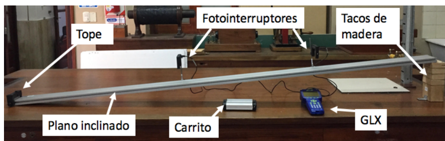
Figura 2. Foto esquemática del sistema experimental: Plano inclinado.
